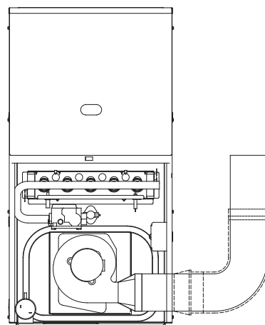
Fig. 13 - Aplicación de flujo descendente: codo de ventilación hacia arriba y luego hacia la derecha
