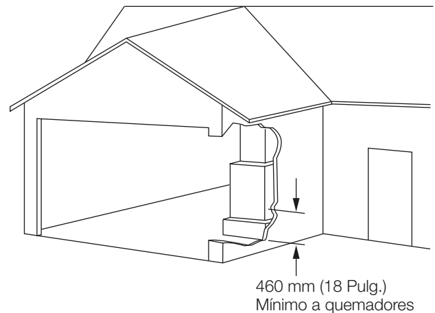
Fig. 4 - Instalación en lavadero / sala de máquinas
