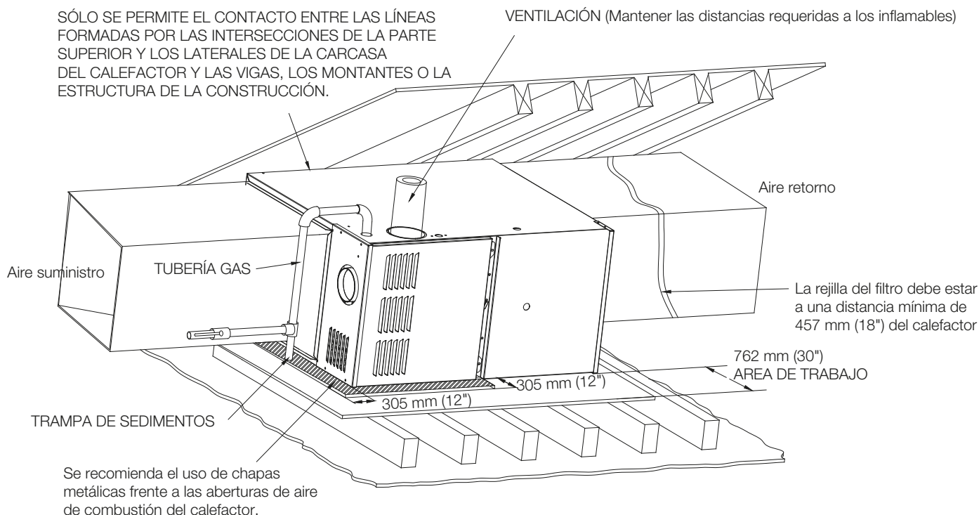
Fig. 11 - Instalación típica en ático
