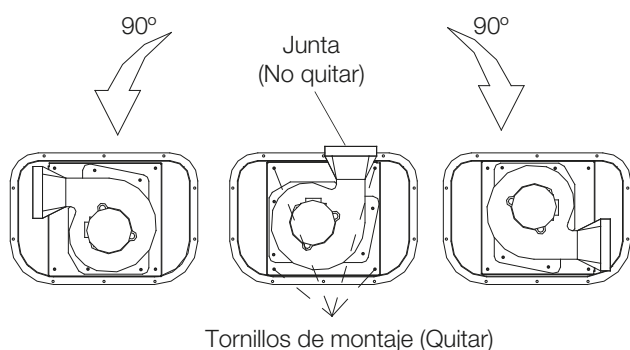
Fig. 20-1 - Inductor de aire de combustión
