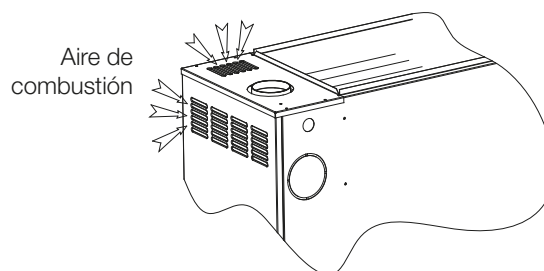
Fig. 21 - Ruta del flujo de aire de combustión a través de la carcasa del calefactor hasta la caja del quemador
