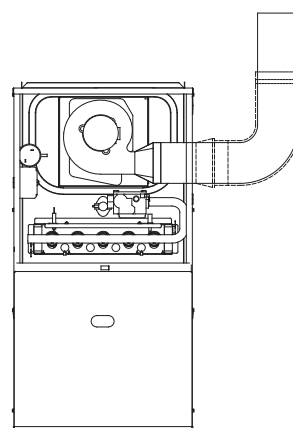
Fig. 18 - Aplicación de flujo ascendente Codo de ventilación derecho
